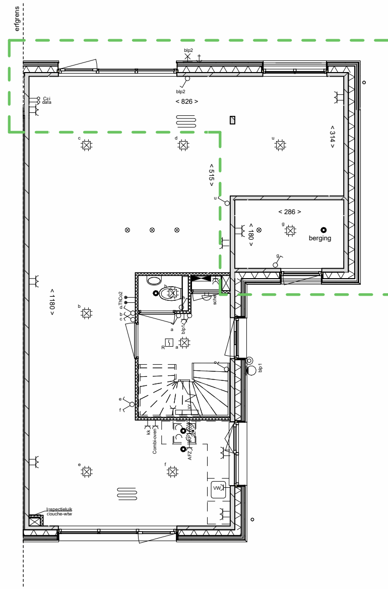
begane grond
