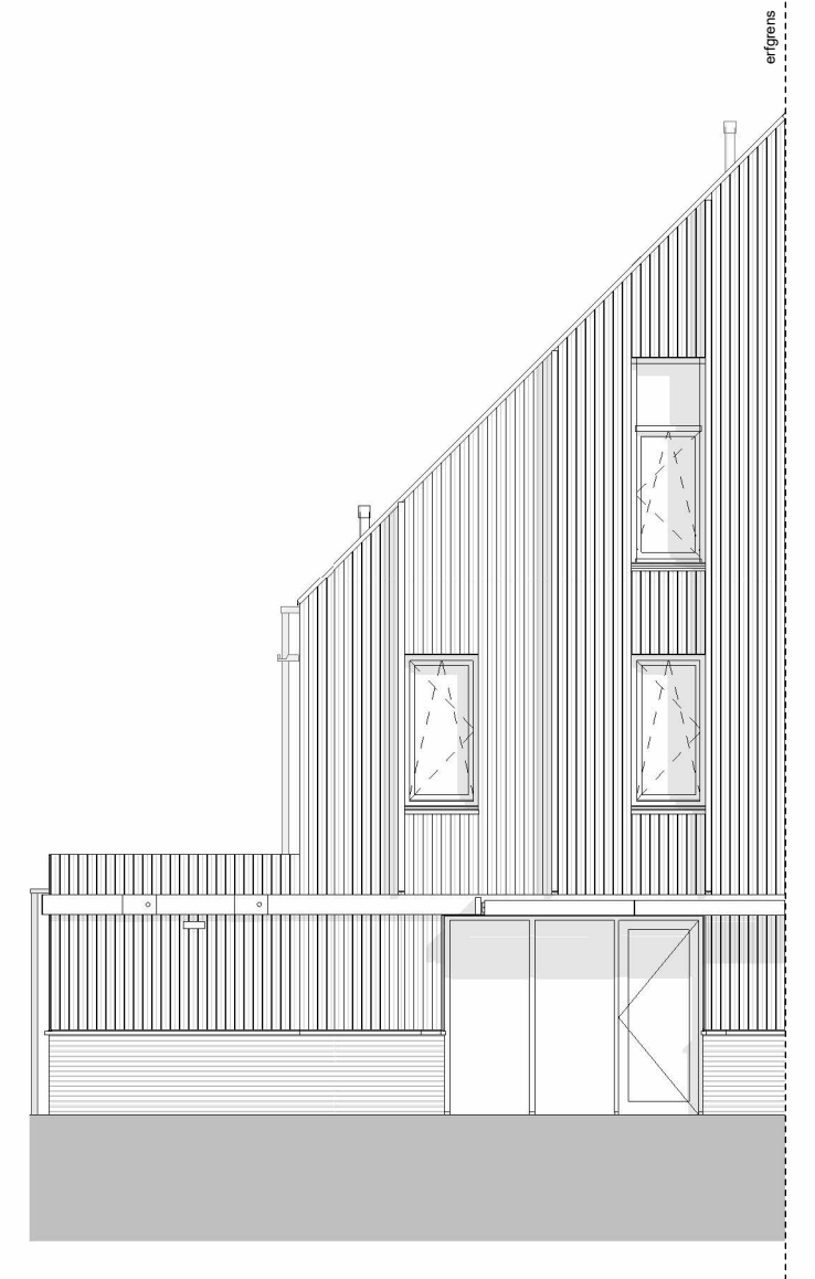
achtergevel (zuidoost)
