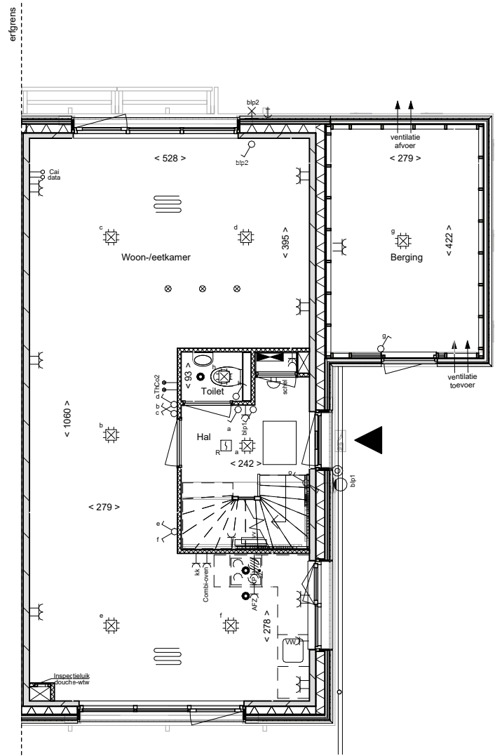
begane grond
