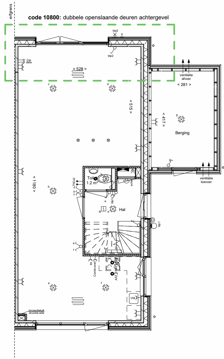
begane grond
