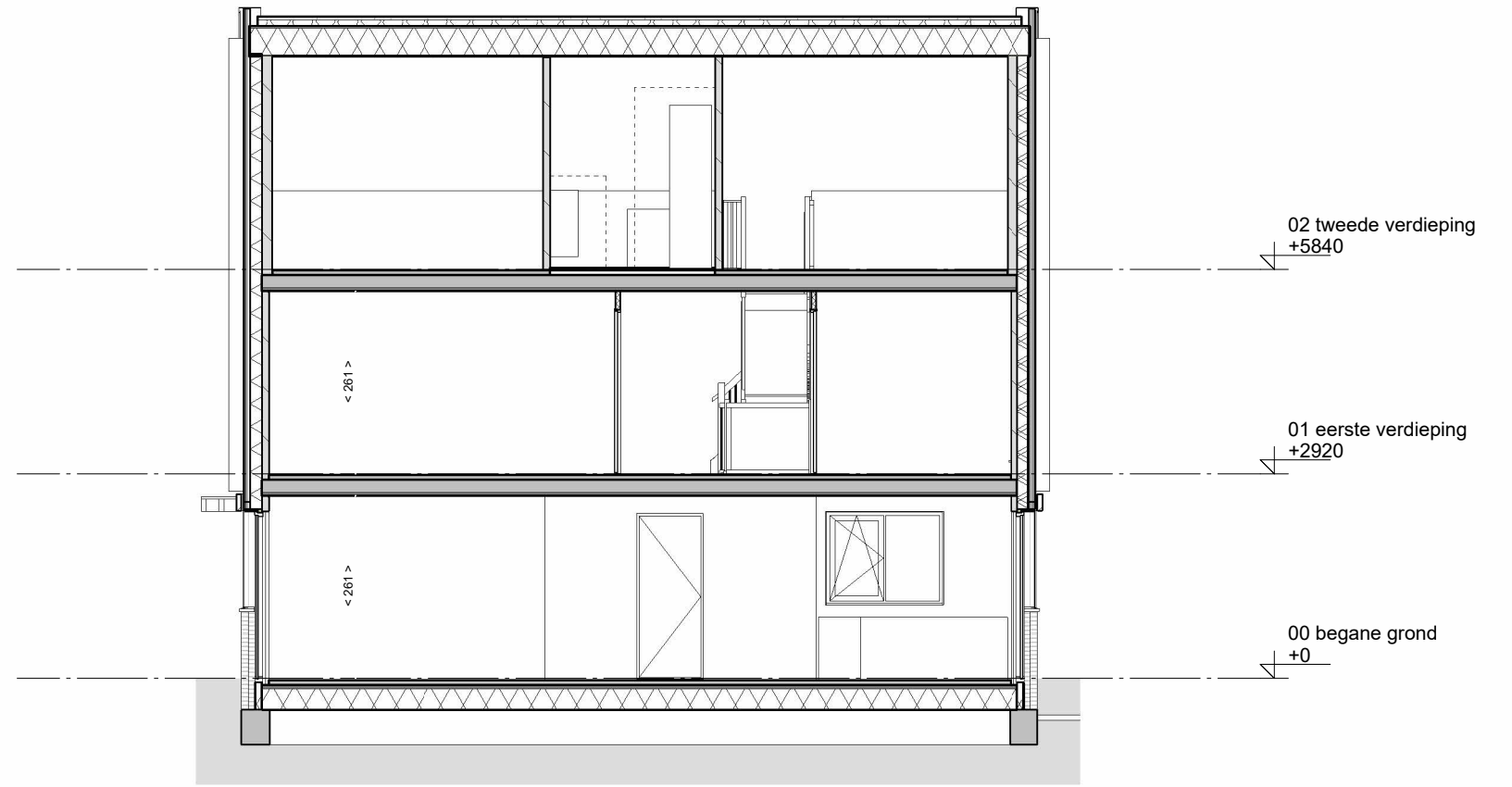
dwarsdoorsnede
