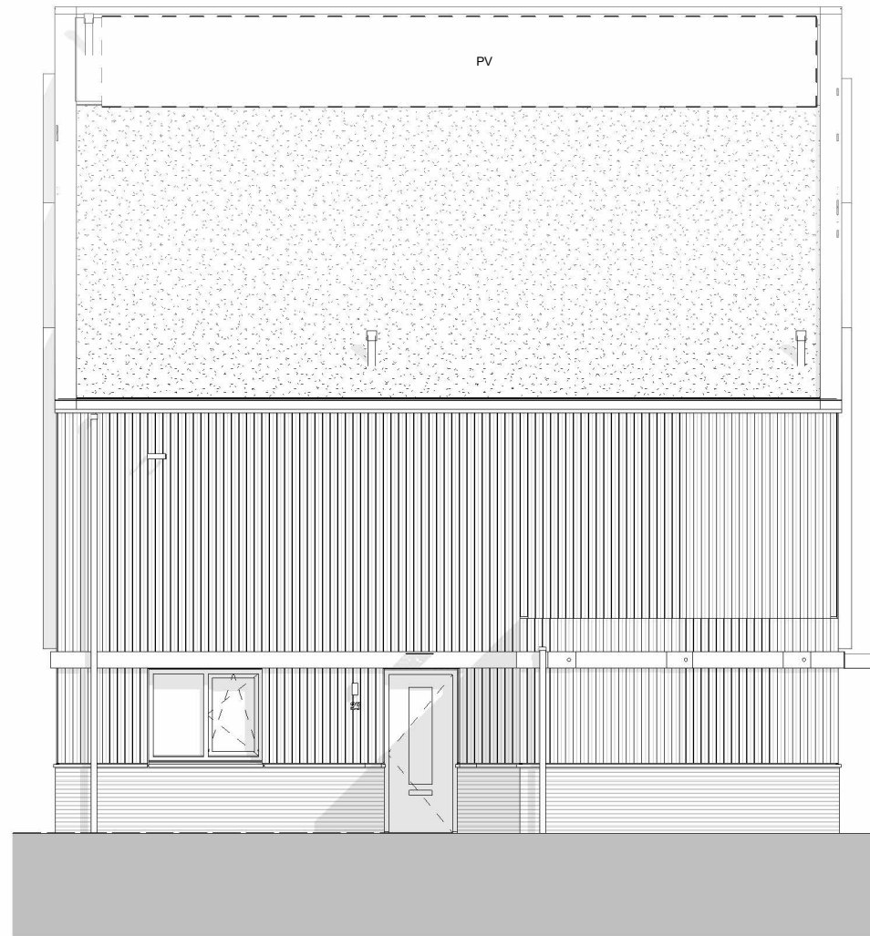
zijgevel (noordoost)
