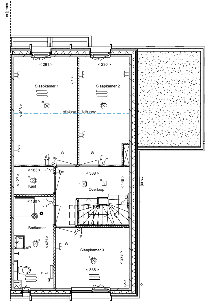
eerste verdieping
