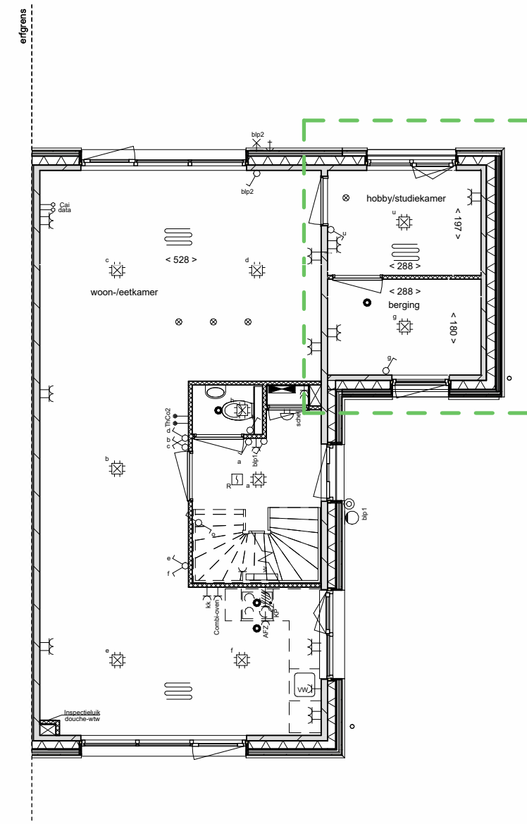
begane grond
