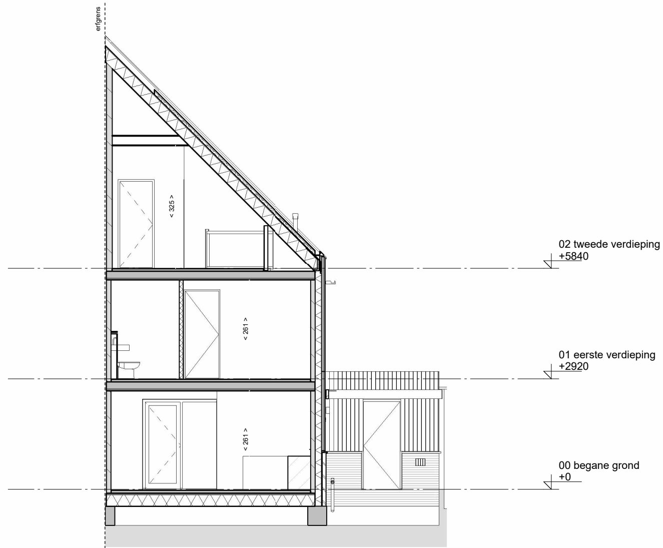
langsdoorsnede
