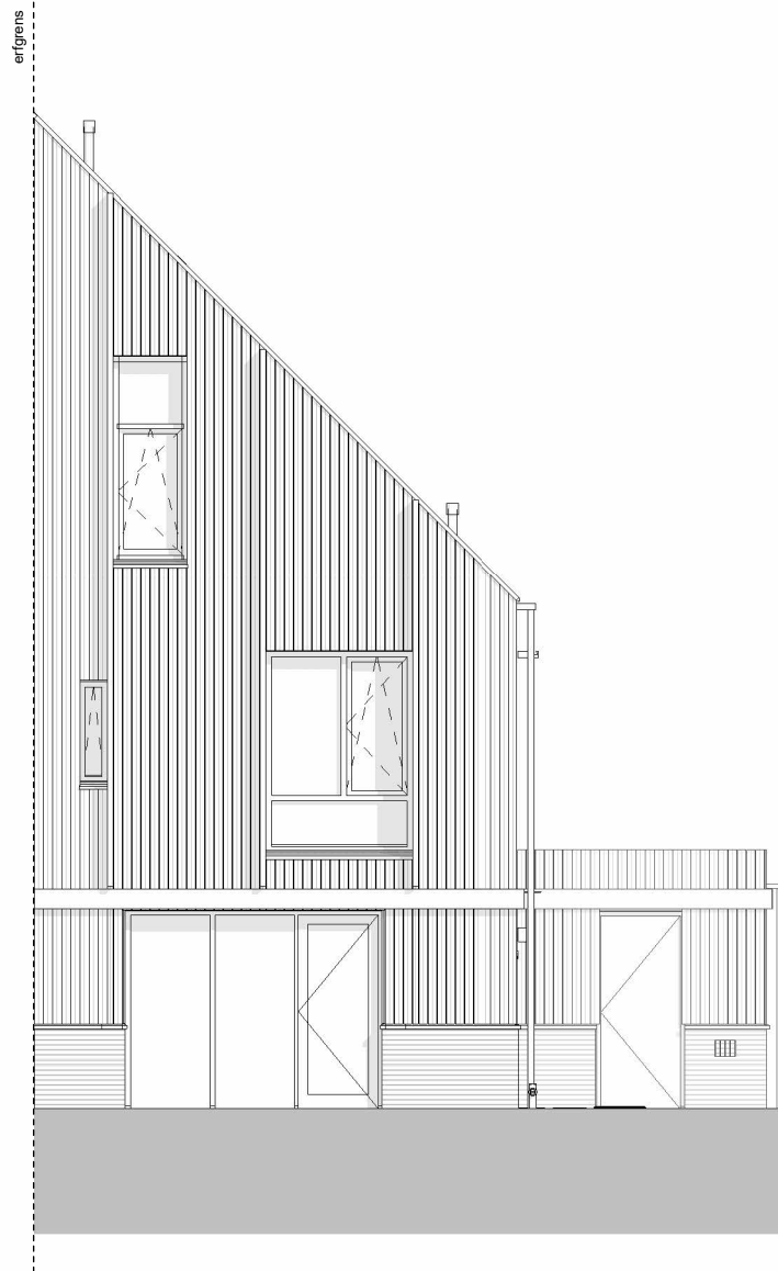
voorgevel (noordoost)
